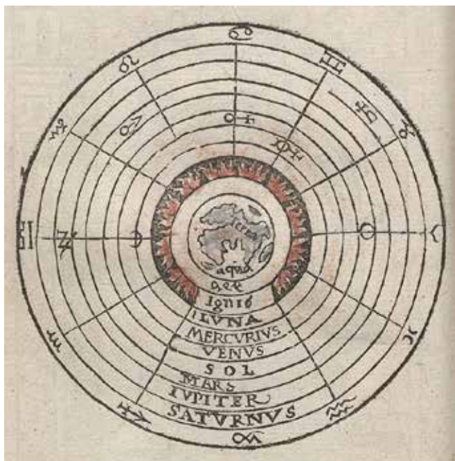
Схема строения Вселенной
