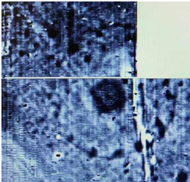
Участок геомагнитной съёмки с круговой структурой – святилище Мергень 5 (VII тыс. лет до н.э.)
