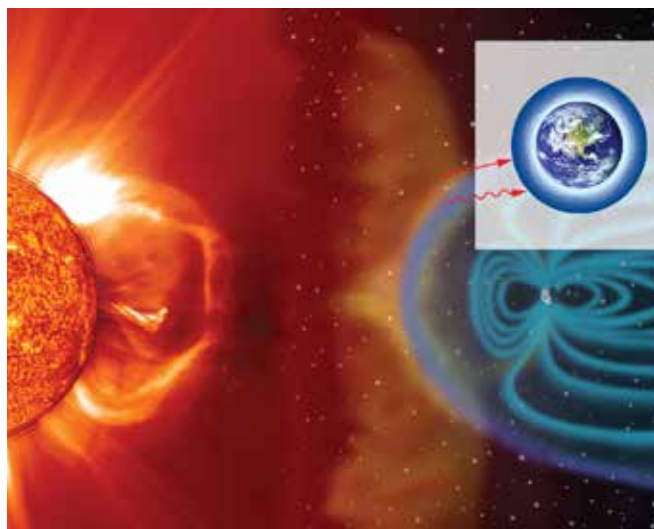
Атмосфера и магнитосфера Земли
